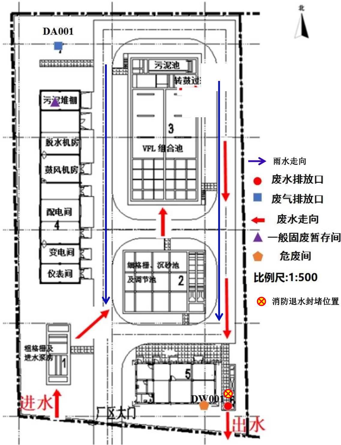
附件 6 雨污水管线图
