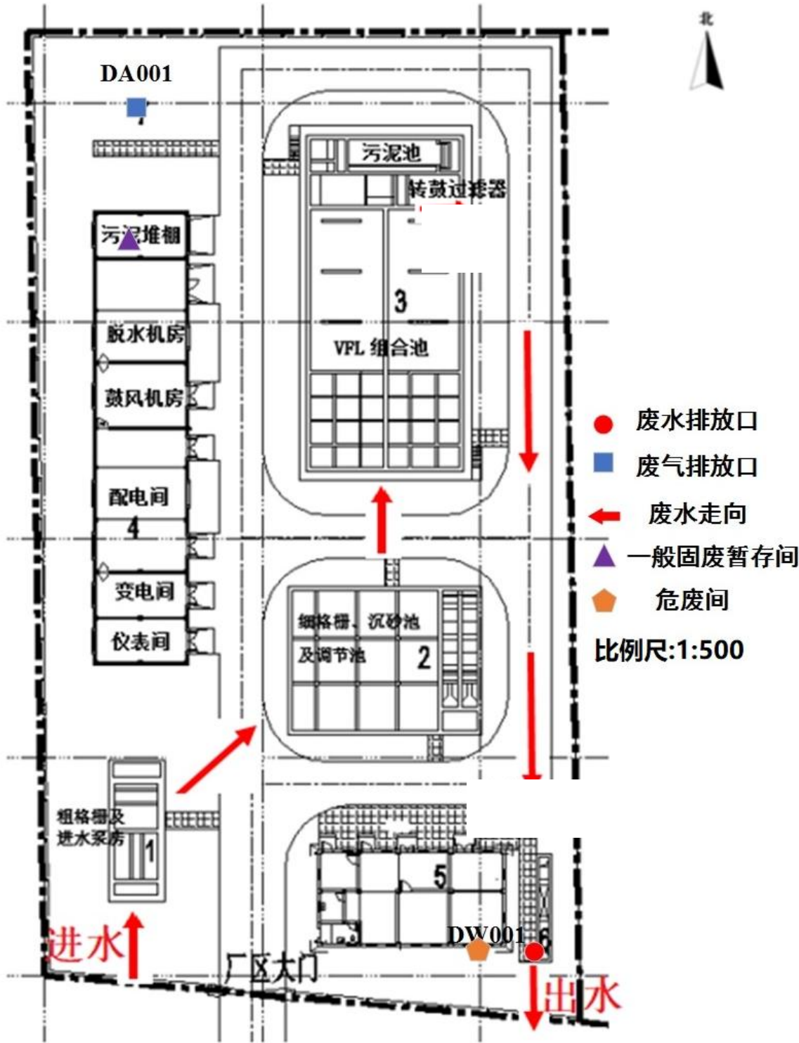
附件 5 厂区平面图
