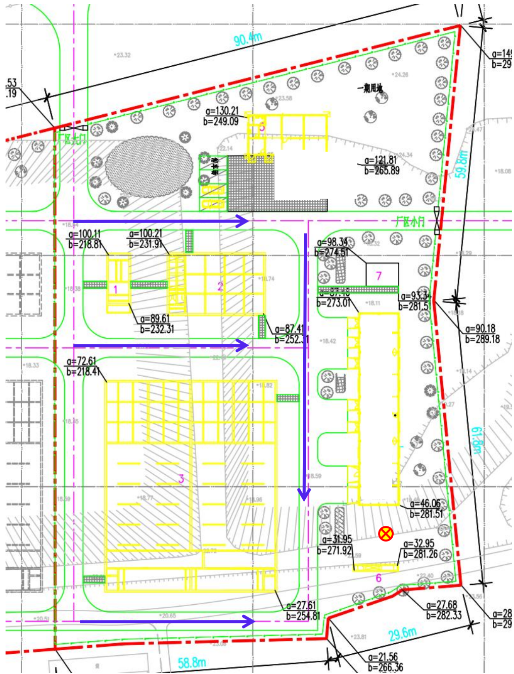
附件 6 雨污水管线图
