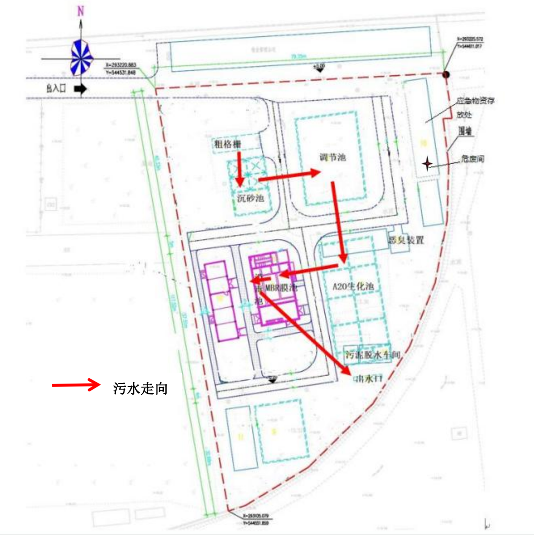
附件 5 厂区平面图
