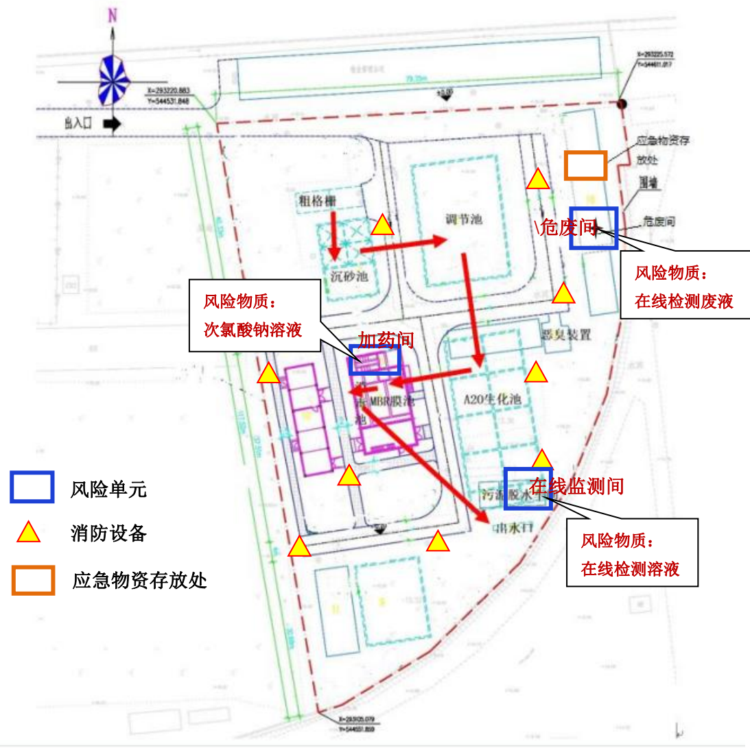
附件 7 应急物资分布图
