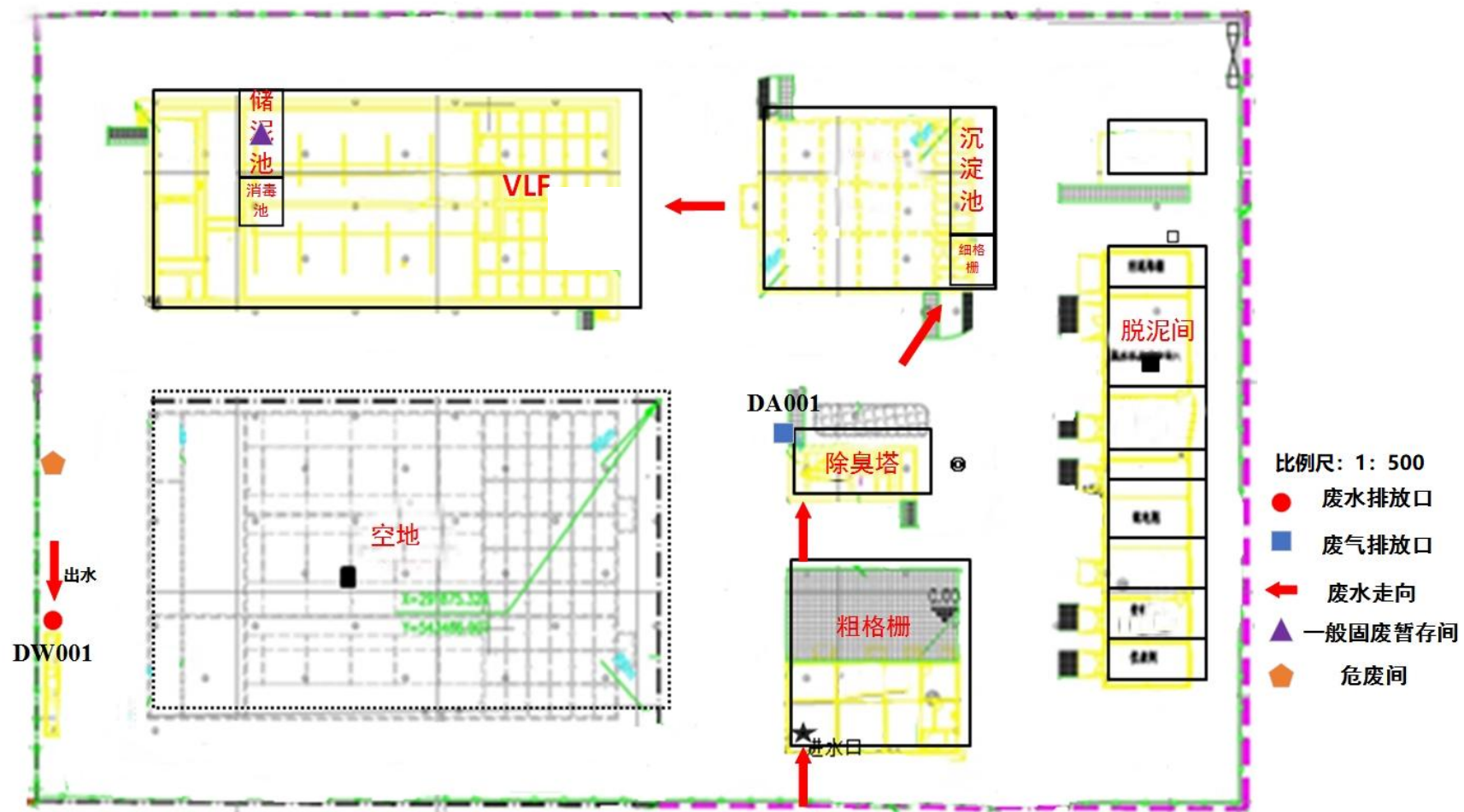
西集镇中心区再生水厂平面布置图
