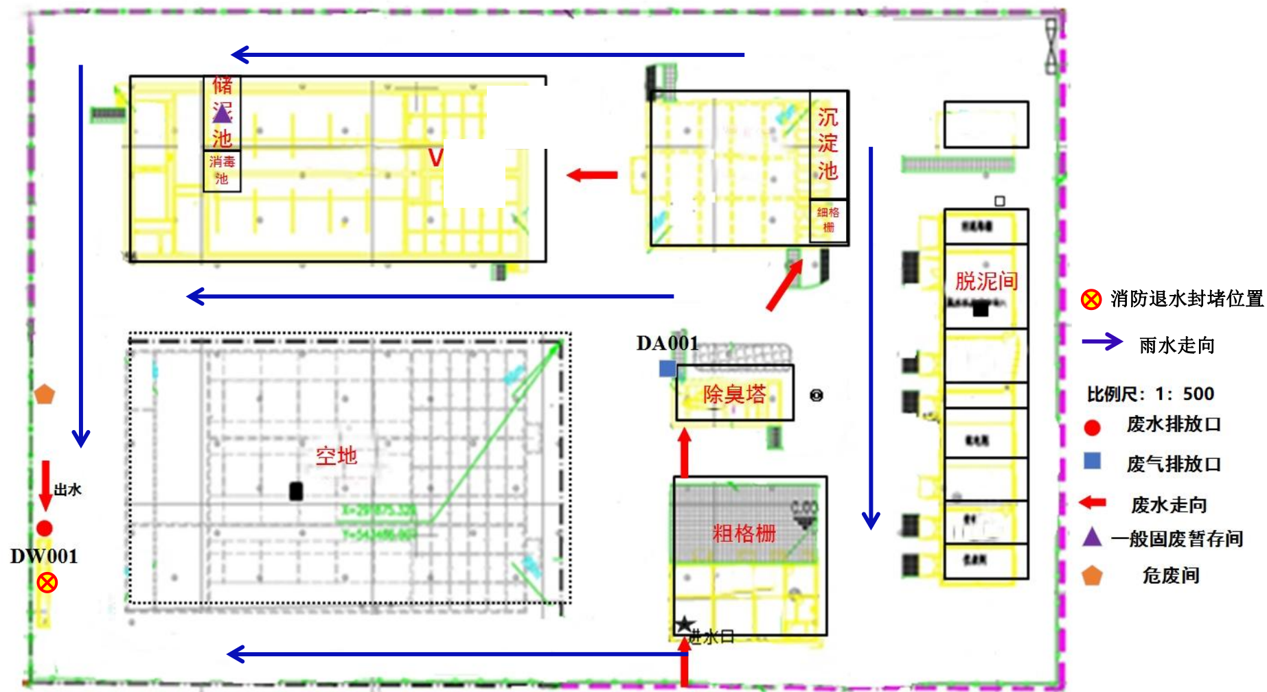
西集镇中心区再生水厂平面布置图
