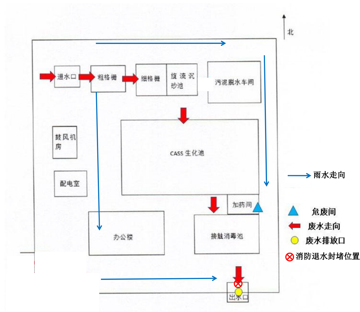
附件 6 雨污水管线图
