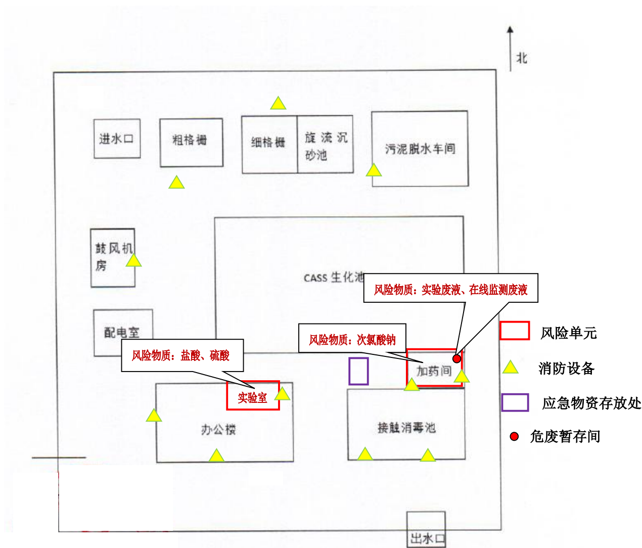
附件 7 应急物资分布图
