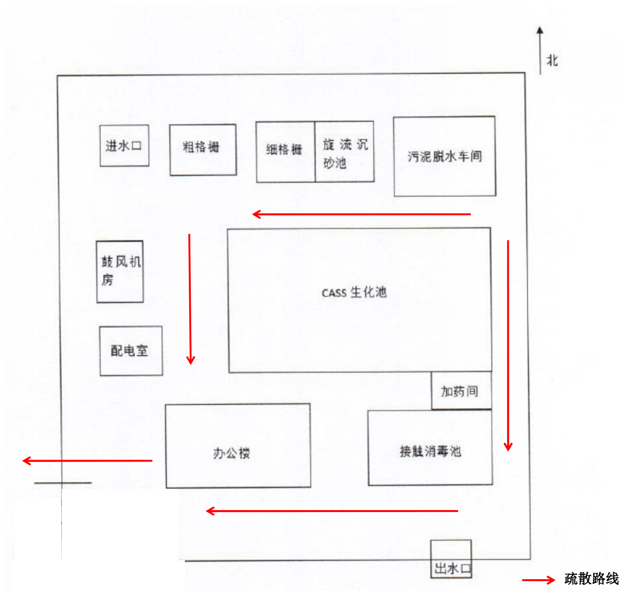
附件 8 人员疏散线路图
