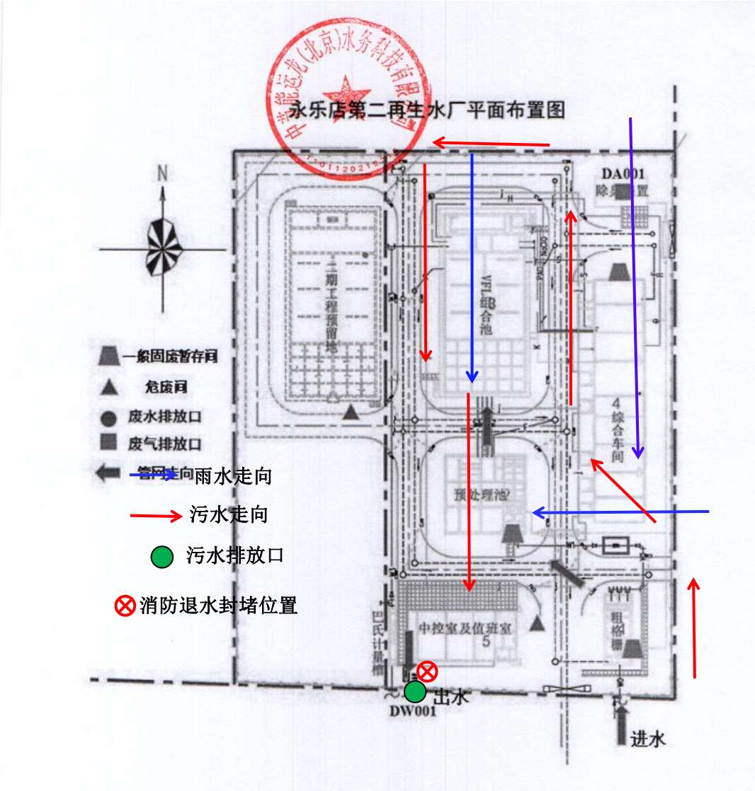
附件 6 雨污水管线图
