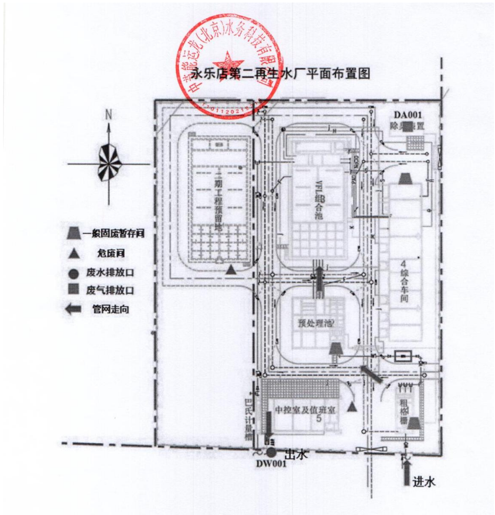
附件 5 厂区平面图
